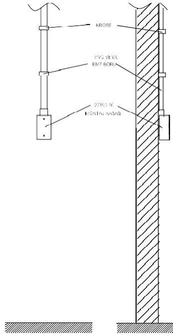
CT2 IZLEME MODULU MONTAJ DETAYI (OLCEKLI DEGILDIR)
