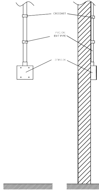
SIREN MODULU MONTAJ DETAYI (OLCEKLI DEGILDIR)
